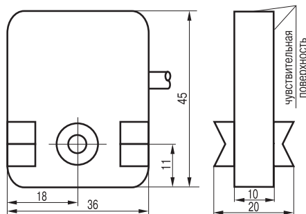
Габаритный чертеж
